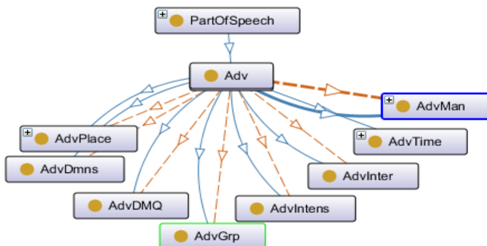
III.2.2.10-Сурет. Қазақ тіліндегі үстеудің онтологиялық моделі.
