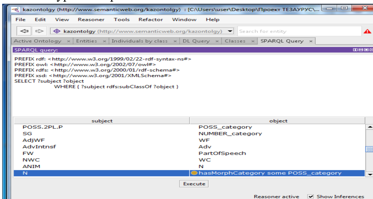
III.3.1.11-Сурет. POSS_category (тәуелдік жалғауы) морфологиялық
