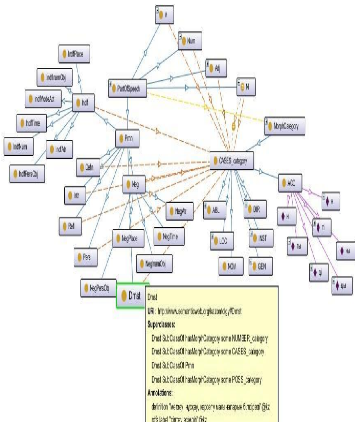
ІІІ.2.2.6-Сурет. Есімдіктің онтологиялық моделі.
