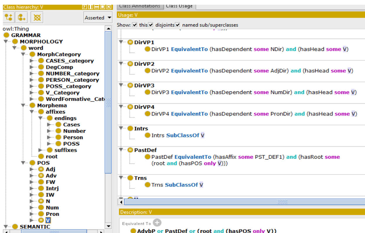
III.2.2.9-Сурет. Етістіктің индивидтерді және сөзтіркестерін байланыстыратын кейбір қасиеттері.
