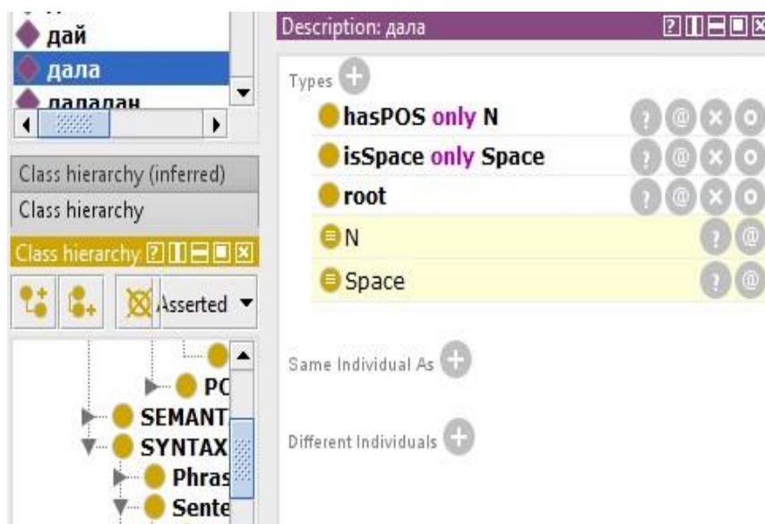
III.3.1.7-Сурет. Онтологияда «дала» сөзінің кеңістіктік мәнге ие зат есім екендігі анықталуы.
