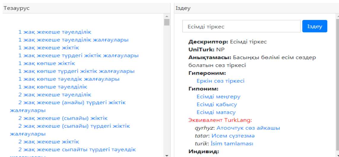
Сурет 4.2- Тезаурус фрагменті, «Есімді тіркес»
