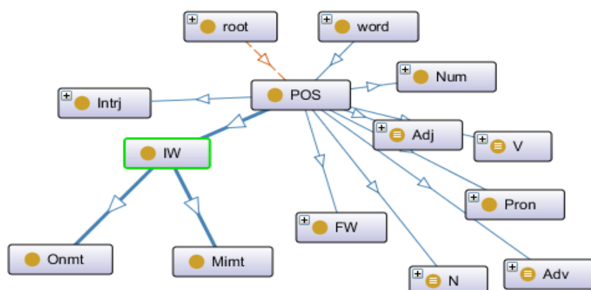
ІІІ.2.2.11-Сурет. Қазақ тіліндегі еліктеу сөздің онтологиялық моделі.
