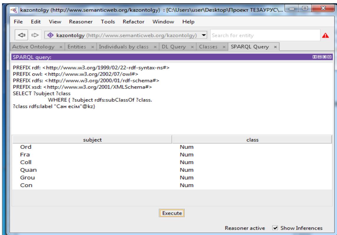
III.3.1.12-Сурет. Num (Сан есім) сыныбының ұрпақтары.
