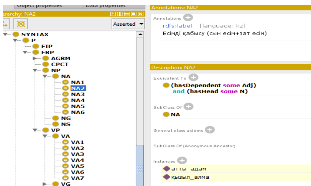
III.3.1.4-Сурет. Сын есім мен Зат есімнің қабысуы.
