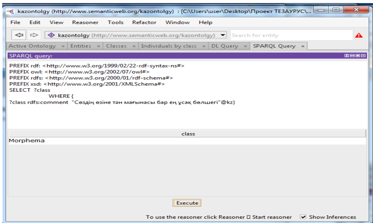
III.3.1.13-Сурет. Берілген түсініктемеге сәйкес кластың мысалы.
