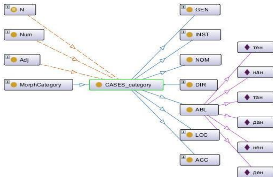
III.2.1.4-Сурет. Шығыс септігінің жалғауларын индивид ретінде көрсету
