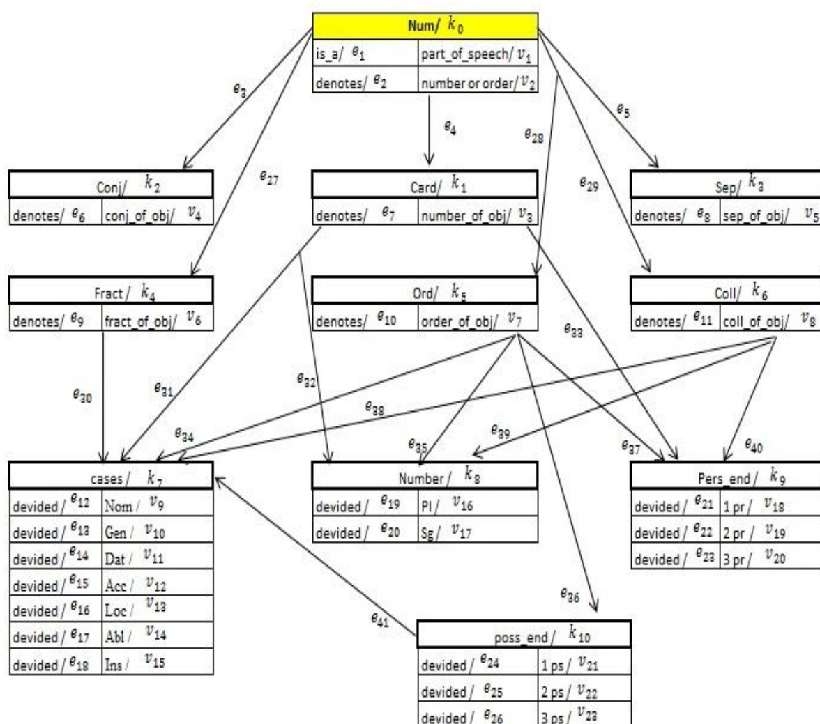
1.2.3-Сурет. Сан есімнің морфологиялық белгілерін семантикалық гиперграф арқылы графикалық бейнелеу
