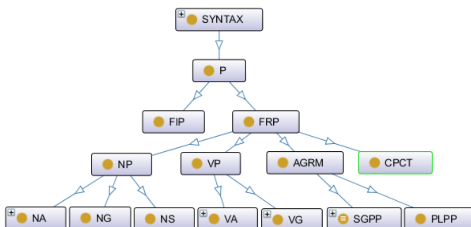
III.3.1.1-Сурет. Қазақ тілі сөз тіркестерінің байланысу түрлері.
