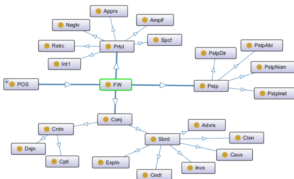
ІІІ.2.2.12-Сурет. Қазақ тіліндегі шылаудың онтологиялық моделі.
