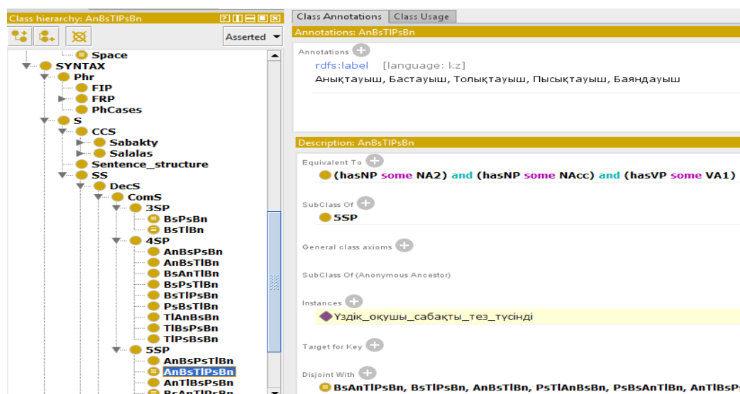
III.3.1.9-Сурет. Қазақ тіліндегі AnBsTIPsBn типіндегі сөйлемнің онтологиялық моделі
