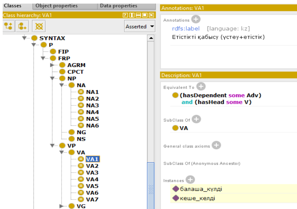
III.3.1.4-Сурет. Үстеу мен етістіктің қабысуы.
